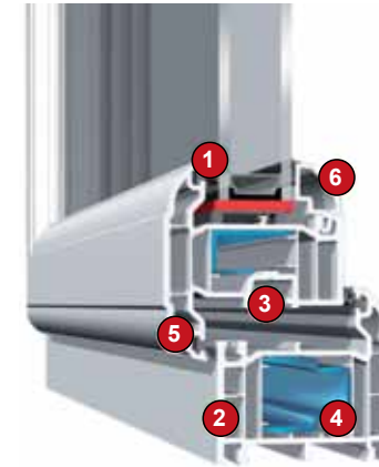
Ovolo O70 System.
